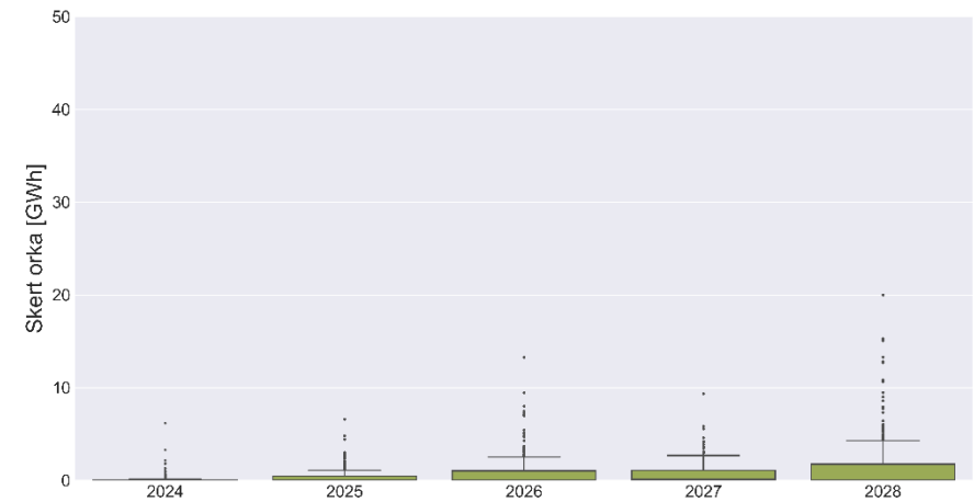
Mynd 14 : Orkuskerðingar almennrar notkunar í sviðsmynd 2
