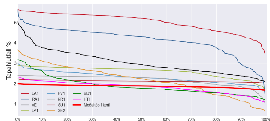
Mynd 31 : Hlutfallsleg töp lína fyrir sviðsmynd 0 í langæislínum
