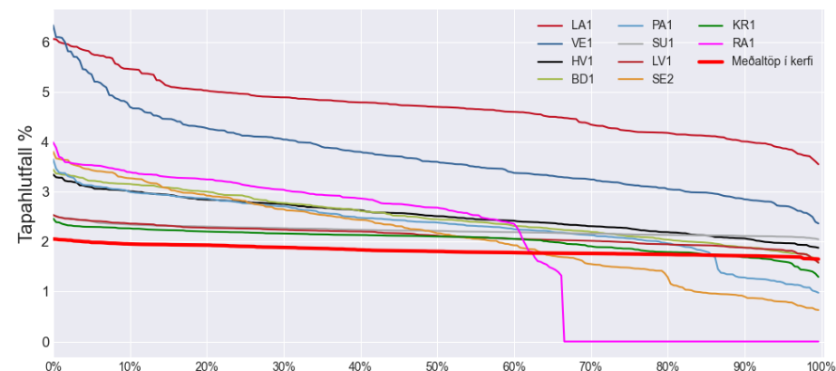
Mynd 33 : Hlutfallsleg töp lína fyrir sviðsmynd 2 í langæislínum
