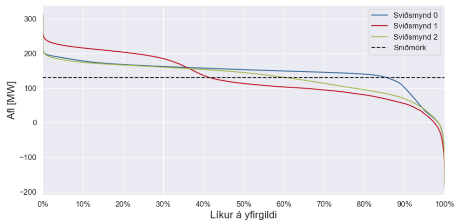
Mynd 28 : Langæislinur flæðis yfir snið IIIb fyrir allar sviðsmyndir
