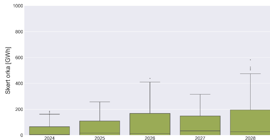
Mynd 8 : Heildarorkuskerðingar í sviðsmynd 2
