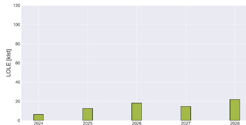
Mynd 21 : LOLE fyrir sviðsmynd 2
