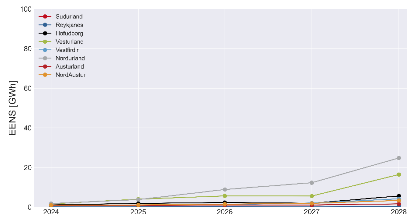
Mynd 16 : EENS eftir landsvæðum fyrir sviðsmynd 0
