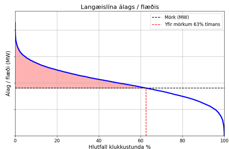
Mynd 37 : Sýnidæmi um langæislínu aflgildis
