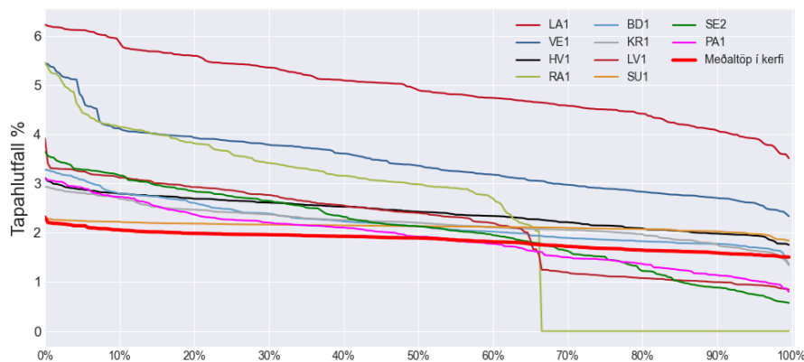
Mynd 32 : Hlutfallsleg töp lína fyrir sviðsmynd 1 í langæislínum
