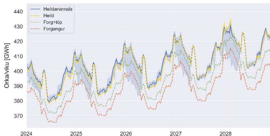
Mynd 5 : Framboð orku samanborið við eftirspurn - sviðsmynd 2
