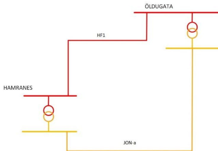
Mynd 3.5.2-1. einlínumynd af flutnings- og dreifikerfinu við Öldugötu
