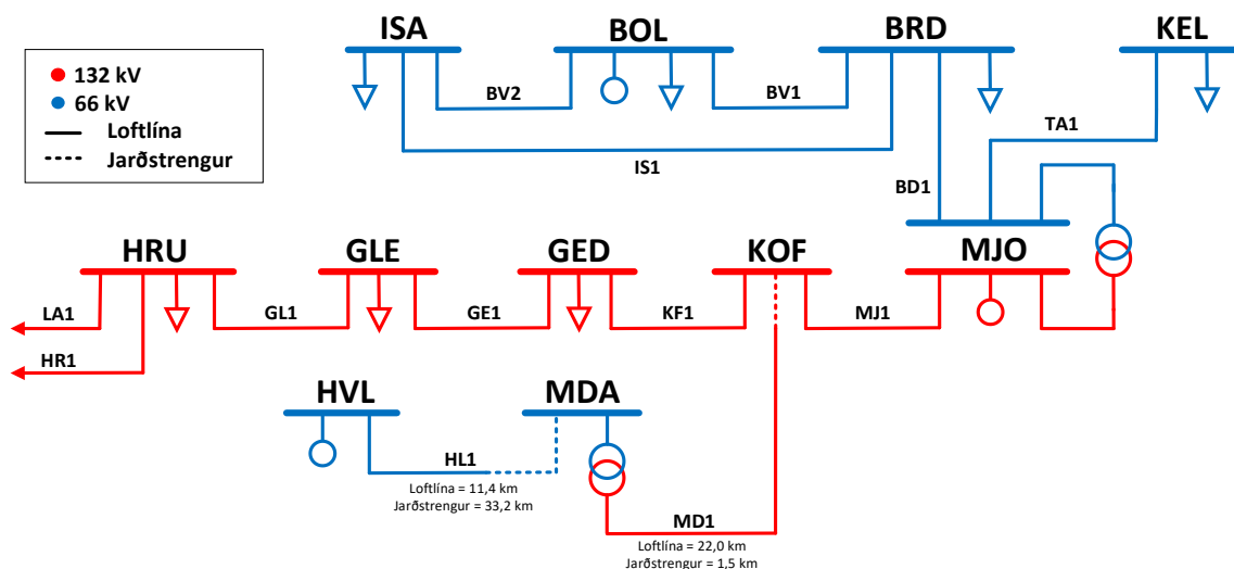
Mynd 3.5.3-1 : Afhendingarstaður í Miðdal – einlínumynd af flutningskerfi Vestfjarða
