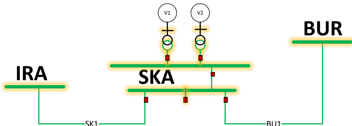
Mynd 3.4.2-1 : SKA - Einlínnumynd af flutningsvirkinu við Hvammsvirkjun
