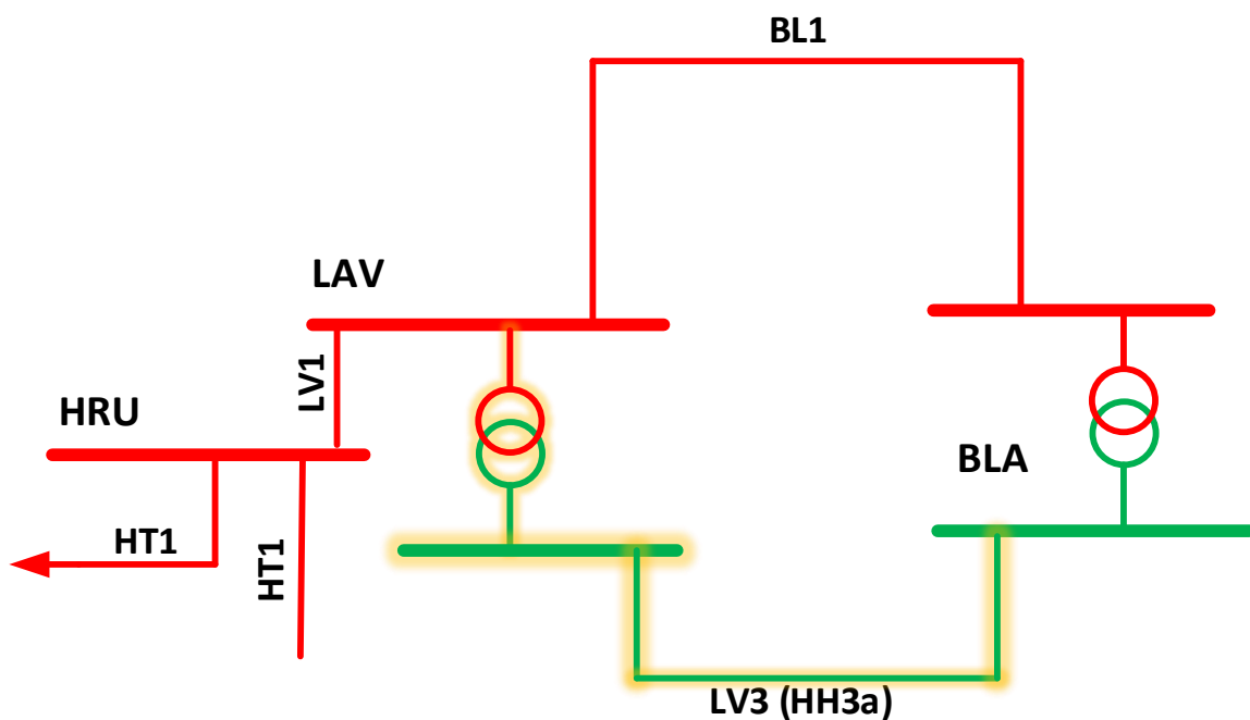
Mynd 3.6.3-2 : fyrsti áfangi HH3 - einlínunmynd með Laxárvatnslínu 3(fyrsta áfanga Holtavörðu-heiðarlínu
