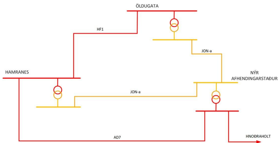
Mynd 3.5.2-5: Einlínumynd af valkosti 2
